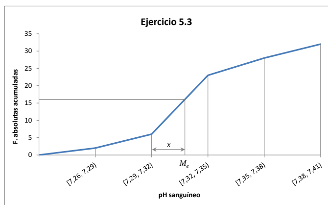
Figura 5.5. Diagrama de frecuencias absolutas acumuladas y cálculo de la mediana para la variable del Ejercicio 5.3.
